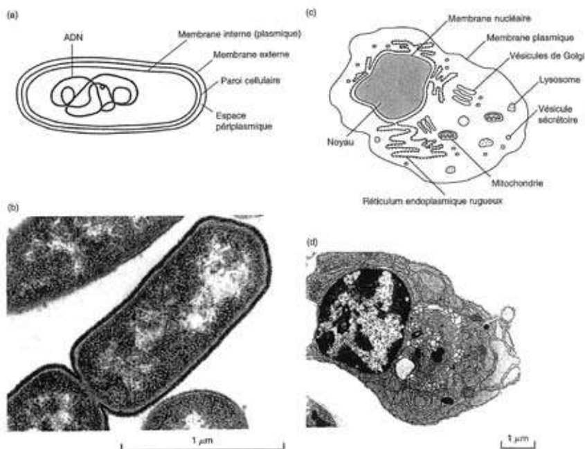
Fig. 2 - Membranes biologiques
