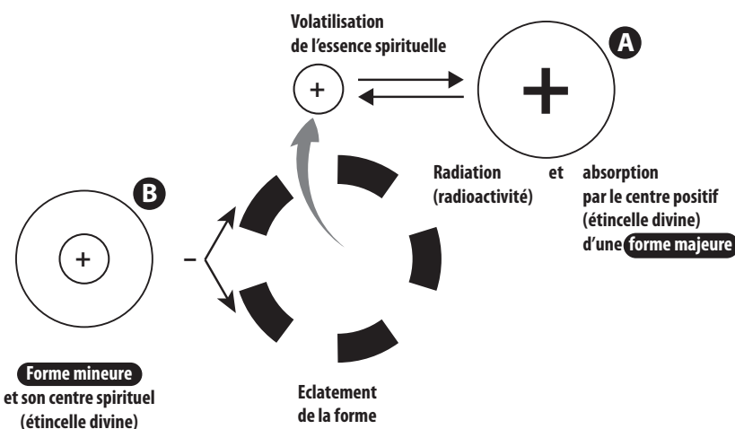
Fig. 3 - Transmutation alchimique
