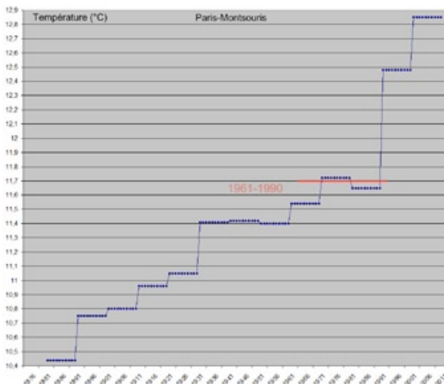
Figure n° 1 : Evolution des températures sur Paris par décennie de 10 ans
